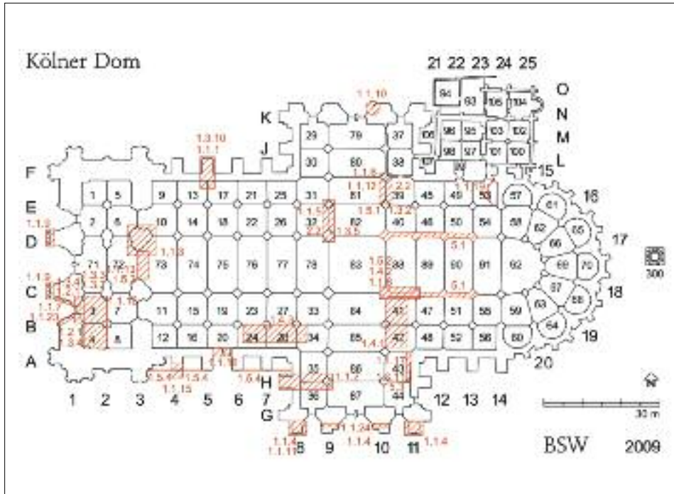
1. Schematischer Grundriss des Kölner Domes mit Eintragung der wichtigsten Arbeiten des Berichtszeitraumes 2008/2009. Die roten Zahlen verweisen auf die Abschnitte des 50. Dombauberichtes.
